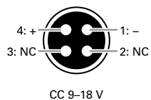
HIROSE 4 broches
