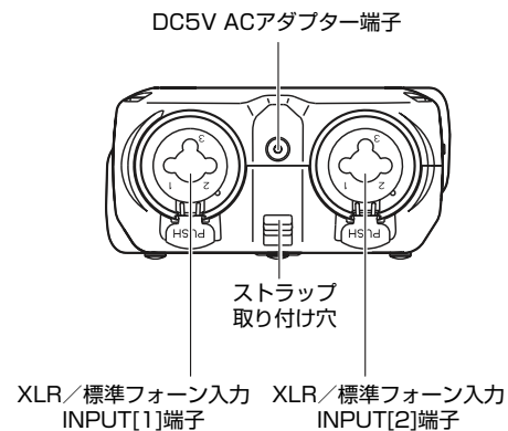
【底面パネル】
